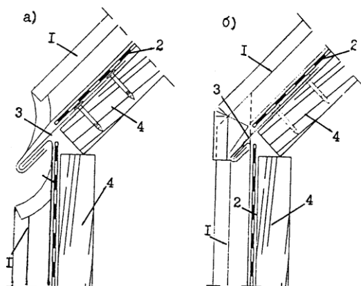
1 – стоячий фальц со скошенными кромками; 2 – подстилающий слой; 3 – карнизный свес; 4 – основание под кровлю
