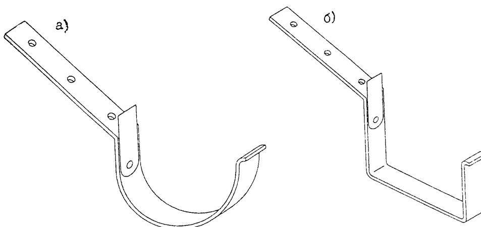
Рисунок 26 – Медный кронштейн для полукруглого желоба (а) и для желоба коробчатого сечения (б)
