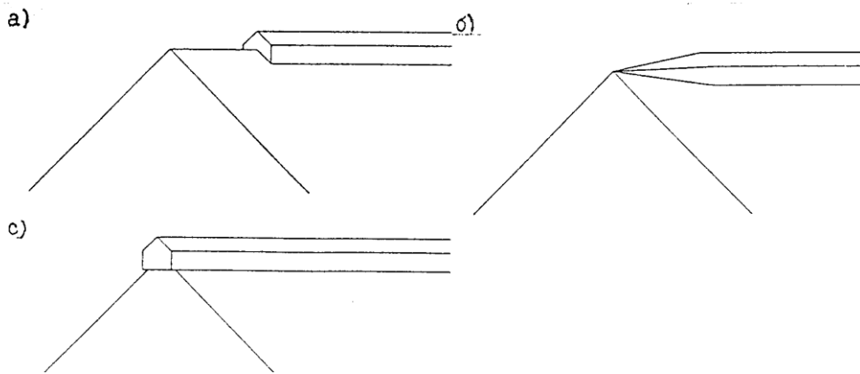
Рисунок 16 – Варианты конечного участка конька на фронтоне
