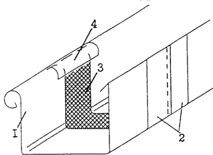
Рисунок 29 – Скользящие соединения шва на стыке полукруглых желобов
