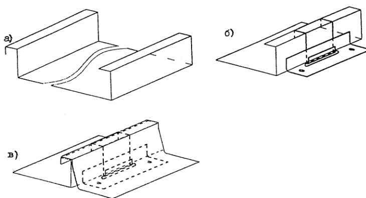
а) изготовление кромок на листе; б) установка кляммера (скользящего кляммера) на основание и кромку листа; в) установка второго листа с отогнутой кромкой образованием двойного стоячего фальца
