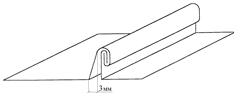
Рисунок 5 – Компенсационный стык
