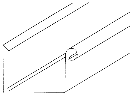
Рисунок 24 – Коробчатый желоб
