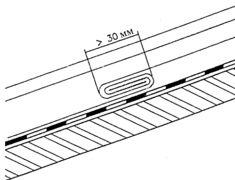
а) одинарный; б) двойной Рисунок 8 – Лежачие фальцы
